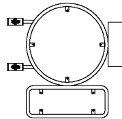
101.56 Brides à gauche, plaque complémentaire et plaquette à droite Briden links, zusätzliche Platte unten und rechts
