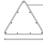
100.28 Support latéral droite pour fixation contre mur Befestigung rechts zur Wandfixierung
