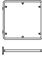
102.15 Fer plats à gauche Flacheisen links
