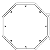
107.14 Fers plats à droite Flacheisen rechts
