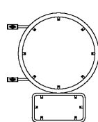
101.107 Brides à gauche et pla- que complémentaire Briden links und zusätzliche Platte unten
