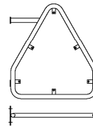
104.07 Fers plats à gauche Flacheisen links
